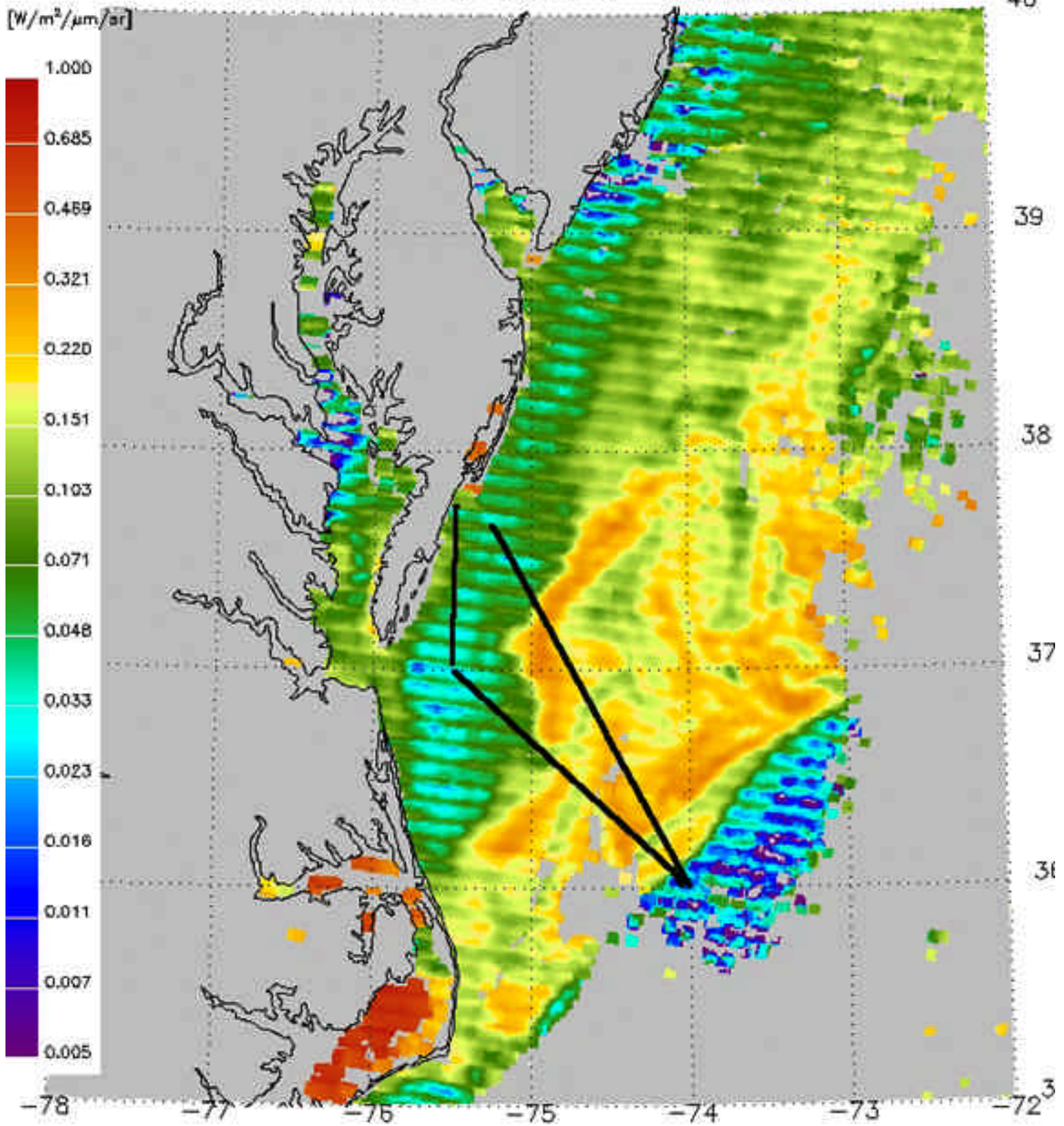
MODIS CHI FLH [ W/m^2/\mu m/sr ] - 03/11/2002
